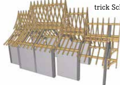
Technische Zeichnung von Patrick Schötz von der neuen Dachstuhlkonstruktion.
